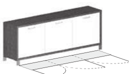
3 dveře VSO22 rozměr: 1800 x 670 x 380
