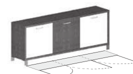
3 dveře VSO24 rozměr: 1800 x 670 x 380
