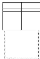
04/R – 2-křeslo bez područek rozkládací 145 × 102/ v. 75-91 ložná plocha 128 × 190/ v. 44
